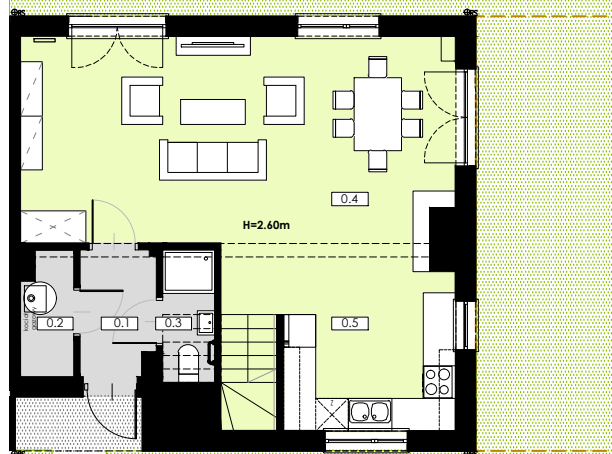
RZUT PARTERU
