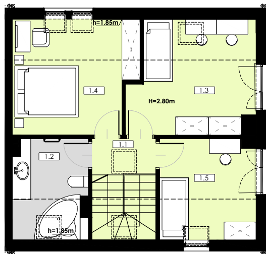
RZUT PIĘTRA
